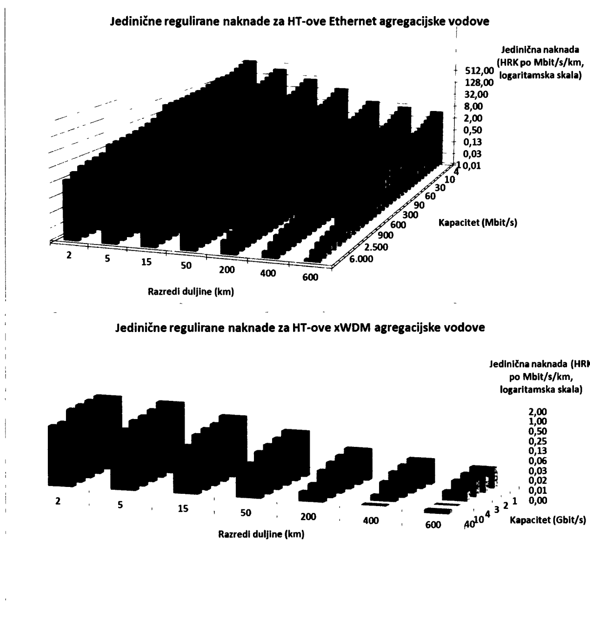
Slika 1-9 – Jedinične naknade za HT-ove regulirane Ethernet i xWDM agregacijske vodove (Mbit/s/km, iznosi prikazani u logaritamskoj skali)
